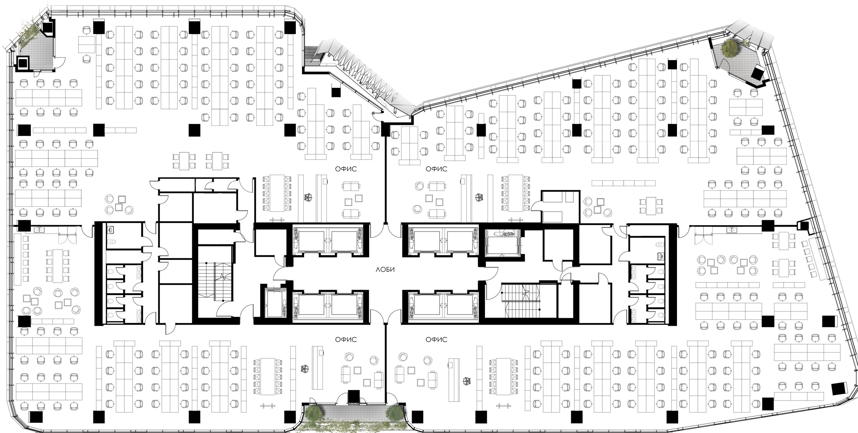
РАЗПРЕДЕЛЕНИЕ ЭТАЖ 6 КОТА +24,60
